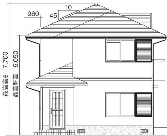
西立面图
