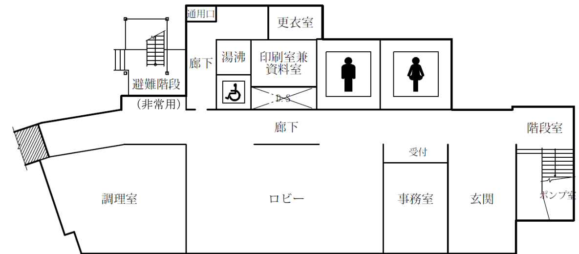
1階平面計画案
