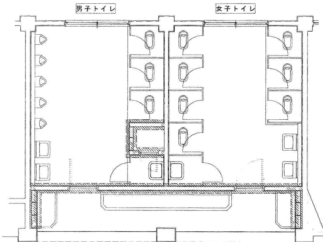
管理・教室棟 2・3 階トイレ（改修前）
