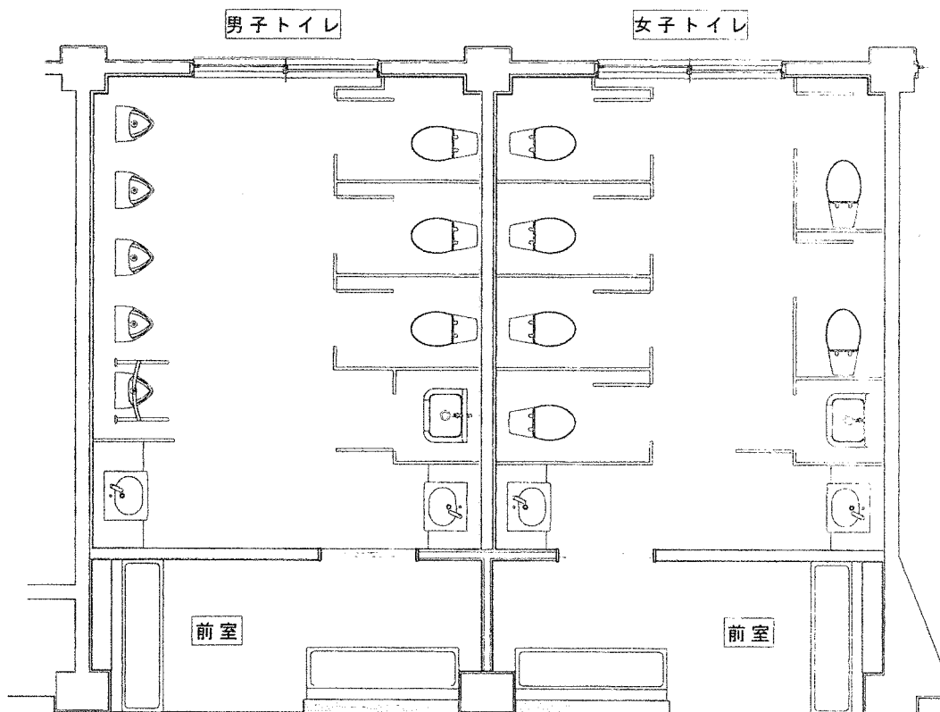
管理・教室棟 2・3 階トイレ（改修後）
