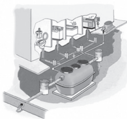
合併処理浄化槽イメージ図
